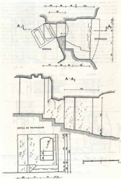
Церковь в Пскове — план и разрез в сечении А-А, сечение А-А1
